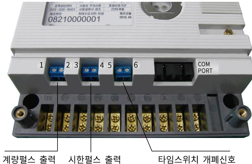
[그림 11] 외부 펄스출력 신호선
