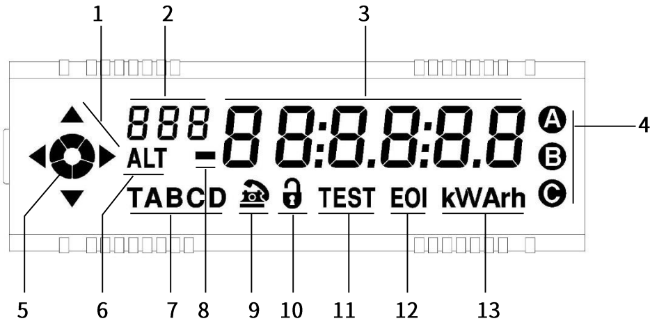
[그림 3] LCD 표시내용
