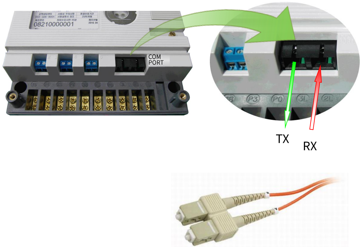
[그림 13] 모뎀 통신포트
