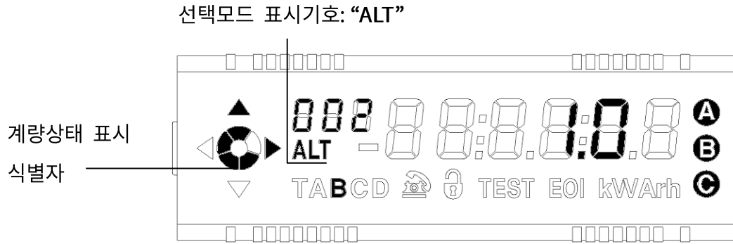
[그림 6] 선택모드(Alt Mode) 표시
