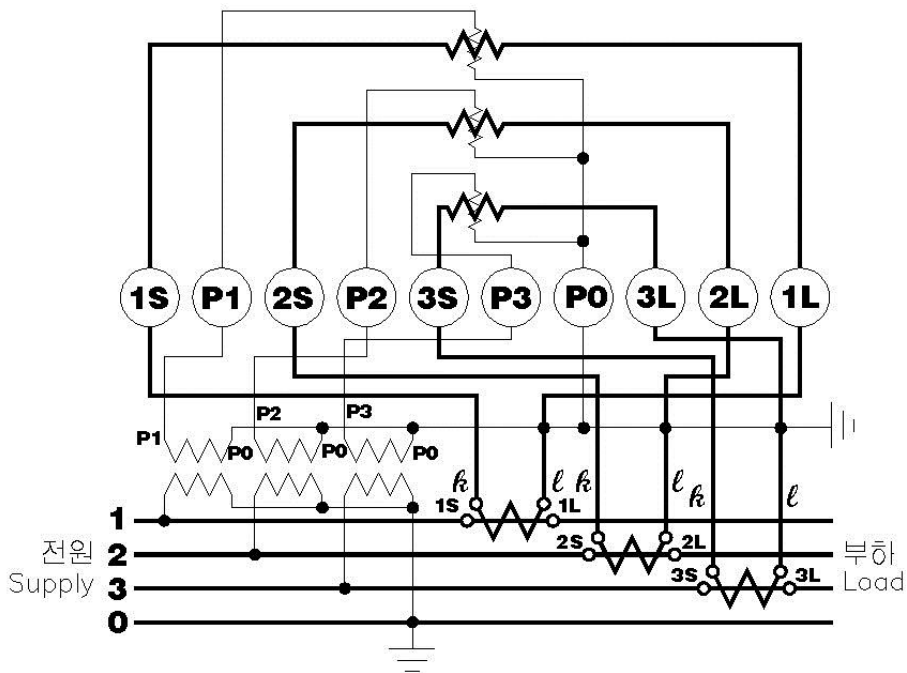
[그림 19] 3상 4선식 결선도
