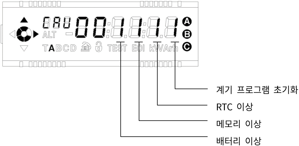
[그림 18] Caution 표시방법
