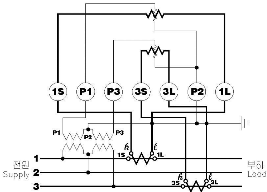
[그림 20] 3상 3선식 결선도
