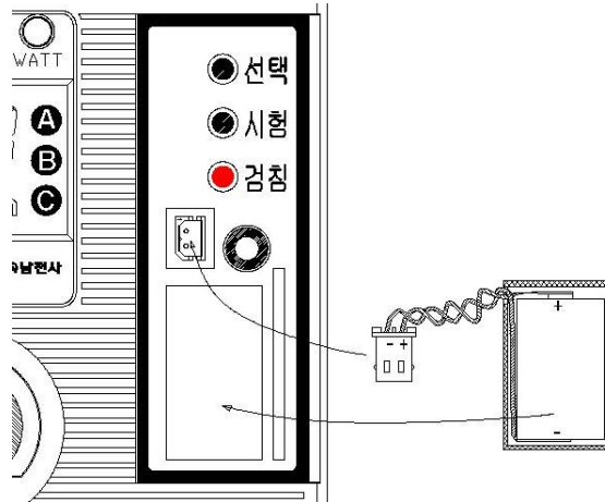
[그림 9] 배터리 부착
