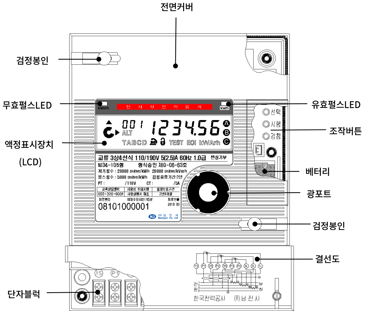
[그림 2] 제품의 외형 및 명칭
