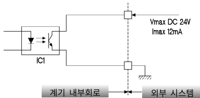
[그림 12] 외부 펄스 출력회로
