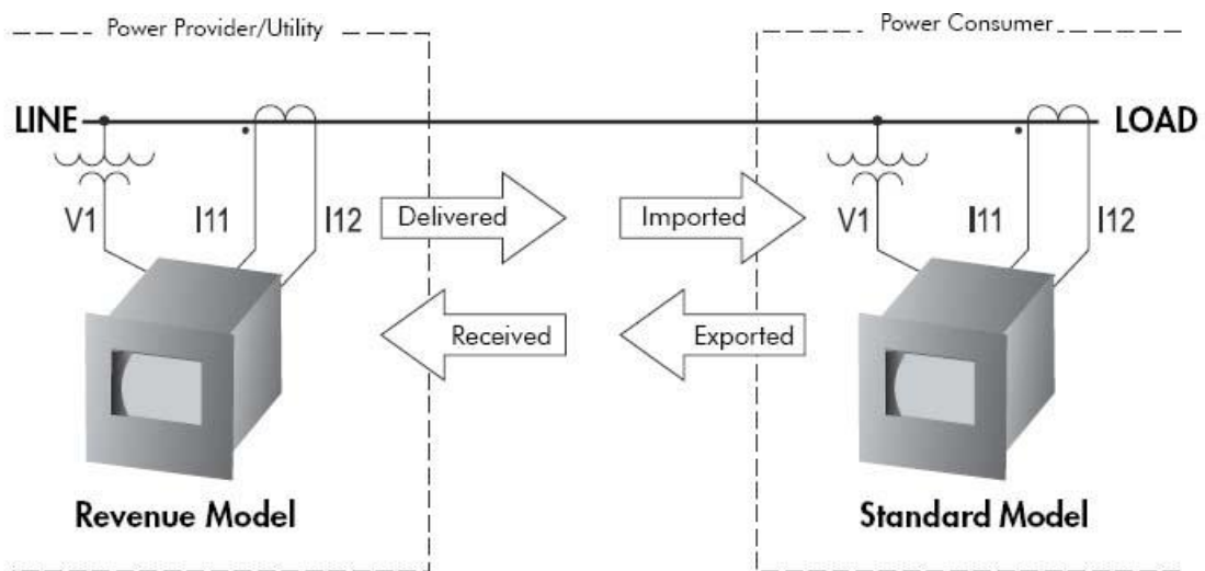
[그림 22] Net metering
