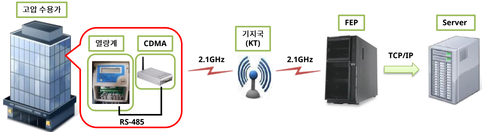
[ CDMA 원격검침 시스템 구성도 ]
